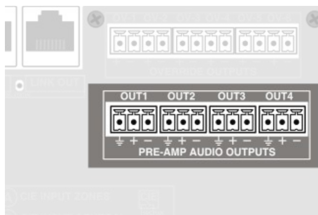
Ilustración 16: Salidas preamplificadas
