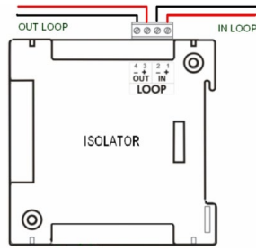
Modulo Aislador: Entrada Loop borne 1 y 2 Salida Loop borne 3 y 4
